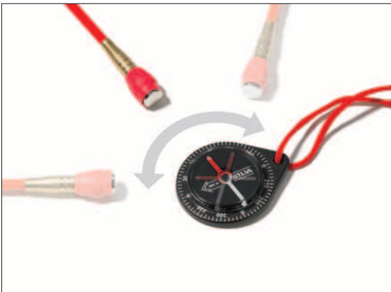
Zur einfachen Ortung bei der Verlegung von Kabeln hinter Wänden – ein Kompass erkennt den auf die Glasfaserstange aufgeschraubten Magneten und erleichtert so die Kabelführung.
